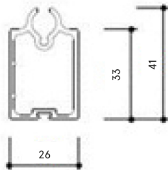
Bottenprofil
