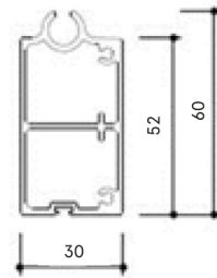
Bottenprofil - dubbel
