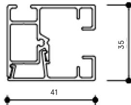
Styrskena - click
