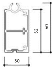
Bottenprofil - dubbel
