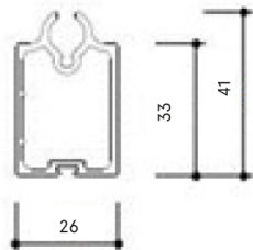
Bottenprofil
