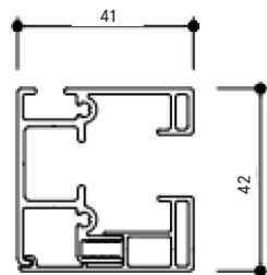
Styrskena - skruv
