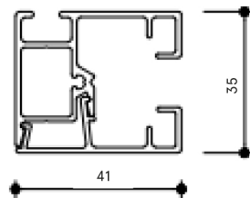
Styrskena - click
